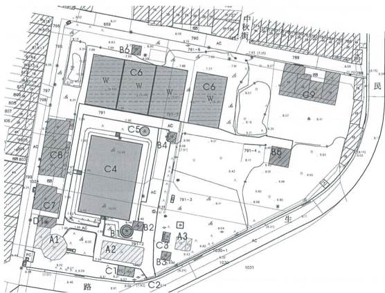
附件 2：北港自來水廠（第一淨水場）配置平面圖
