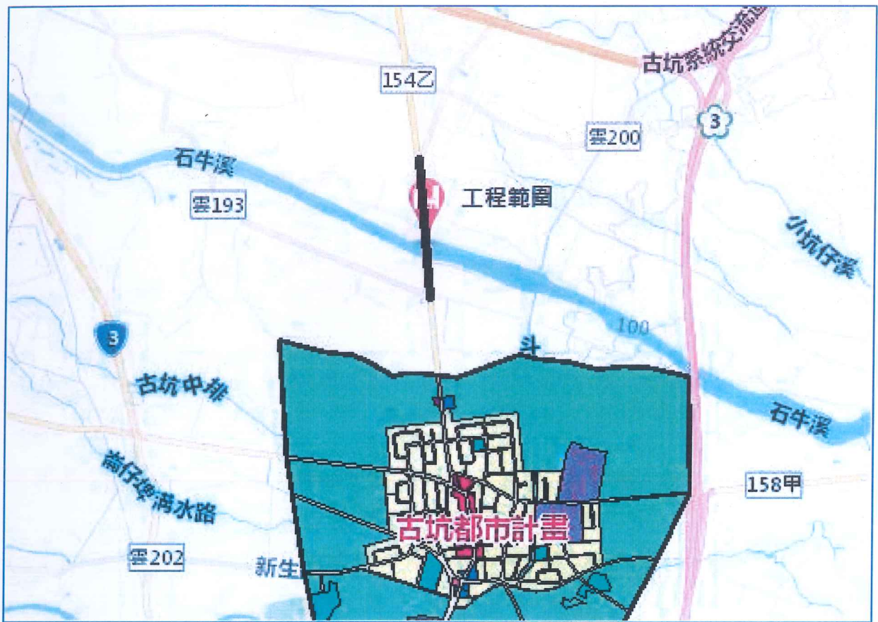
「縣道 154 乙線-水碓南橋改建工程」路線示意圖
