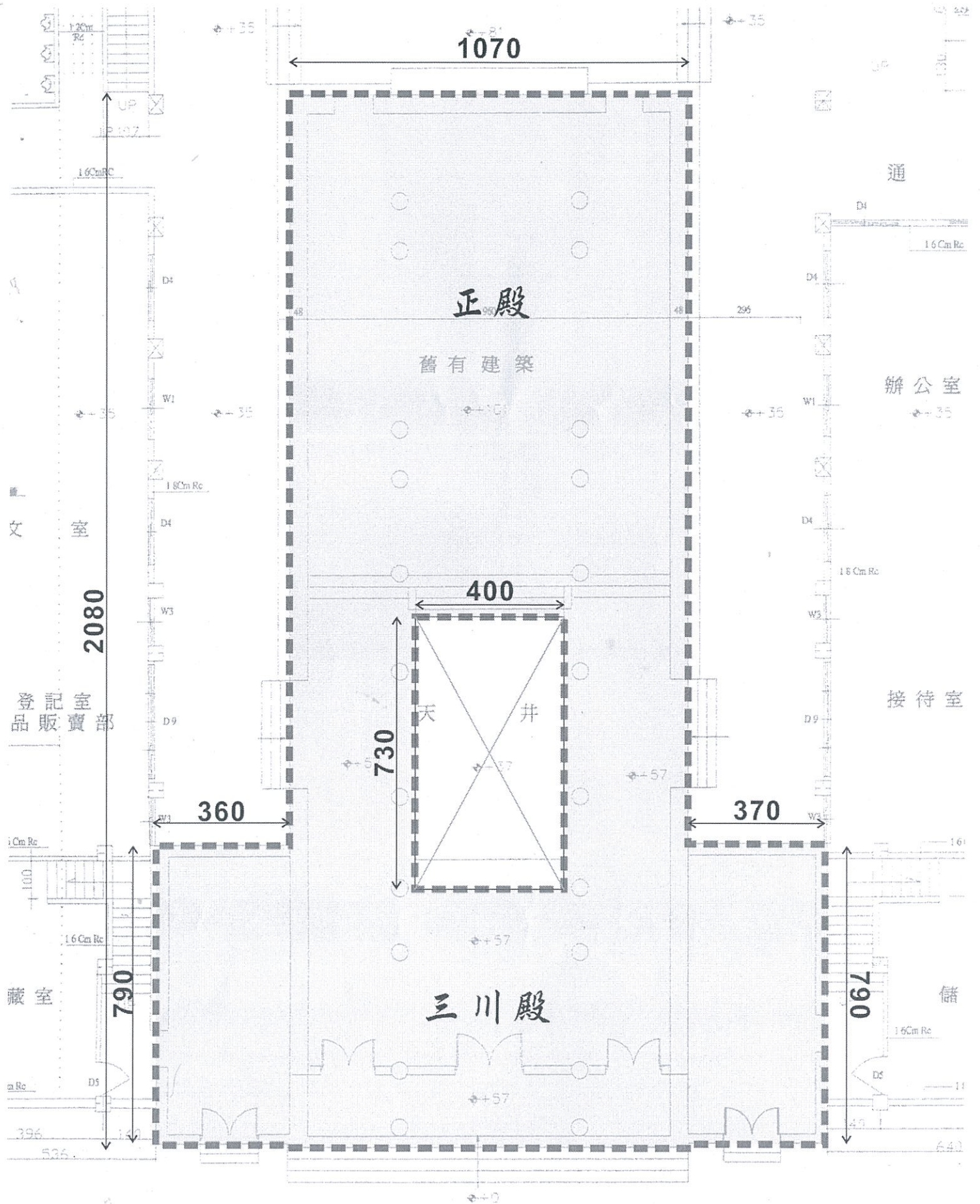
西螺廣福宮 一層平面圖
